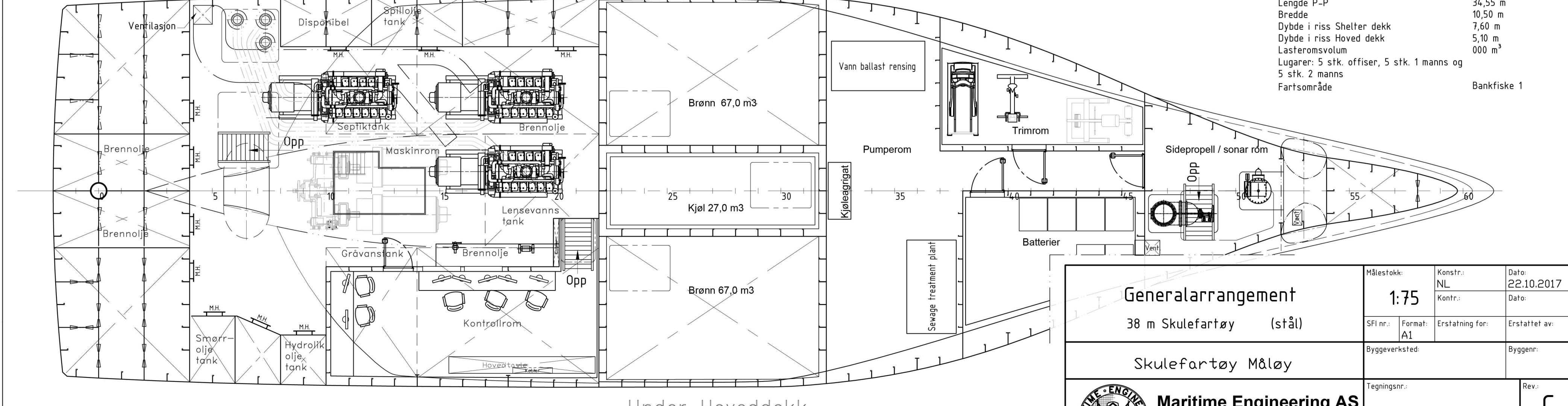
Under Hoveddekk
