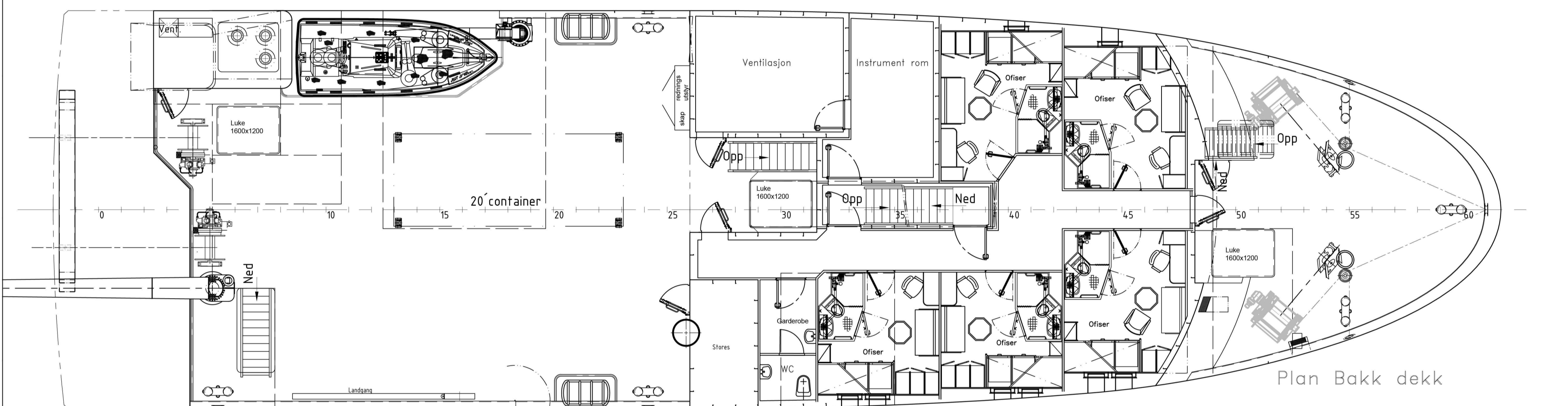
Plan Brodekk
