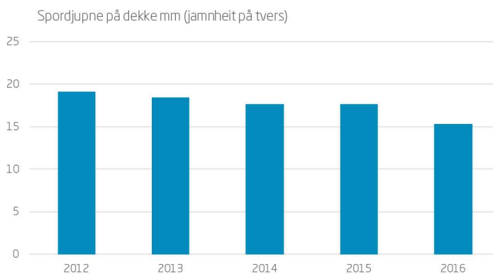
Diagram 18: Spordjupne seier noko om kvaliteten på vegdekket. Auka bruk av midlar i 2012 – 2015 har gitt ein reduksjon i spordjupne. Det er i 2016 ikkje utført målingar på heile vegnettet slik at talet ikkje gir ein korrekt middelværdi. Grunna feil i måleutstyret har vi ikkje data for 2017.
